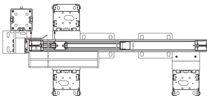
Coupe horizontale
