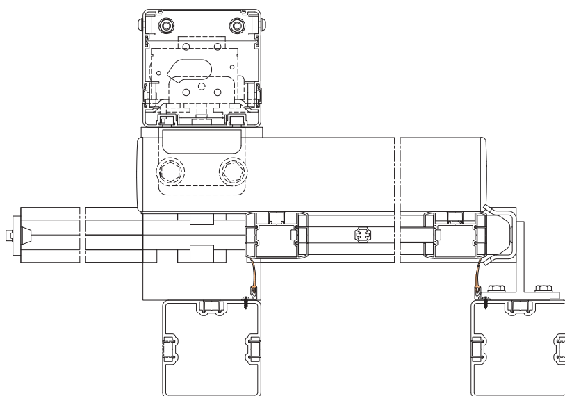
Coupe horizontale
