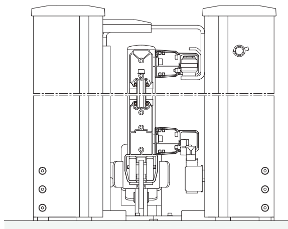
Coupe verticale
