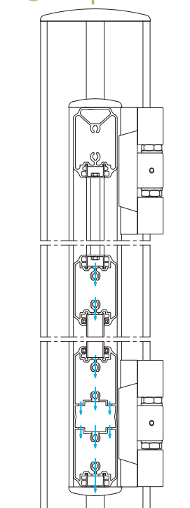
Coupe verticale
